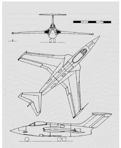
Projet de MS 800 mono réacteur 1954
